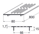
Grile de ventilație
