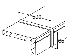
Profile de legătură pentru pervazul ferestrei
