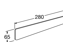
Capace de capăt lateral pentru rebord
